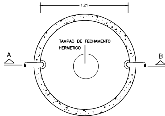
PLANTA BAIXA
