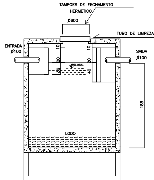
CORTE A-B
